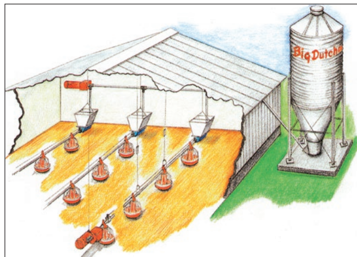
Схема пташника з лініями годування AUGERMATIC
