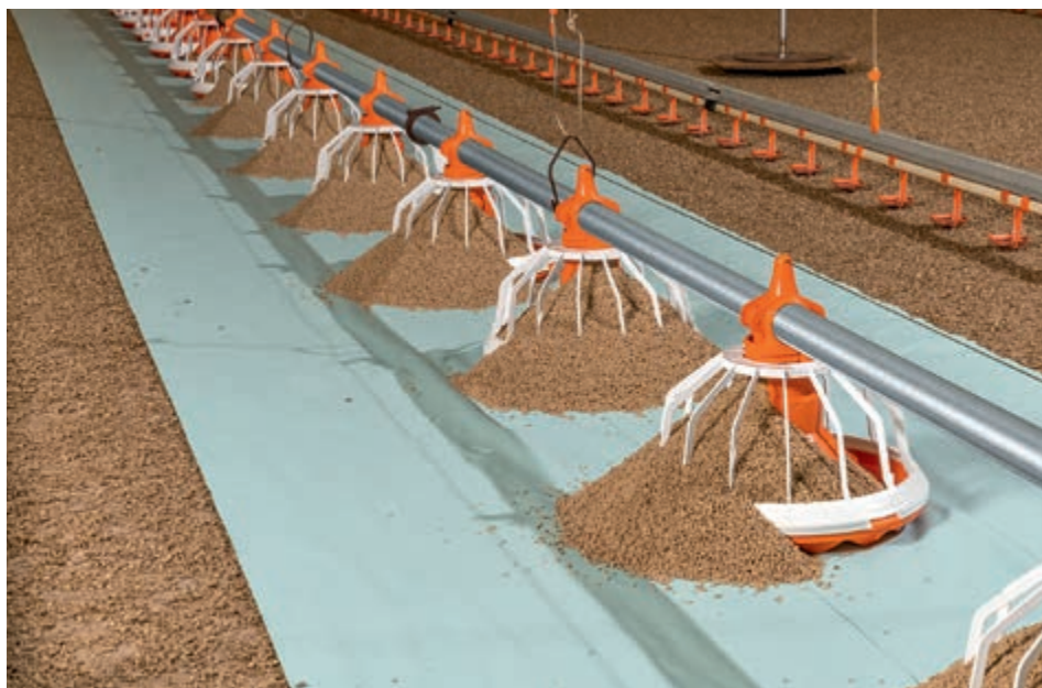
W celu optymalnego startu tuczu piskląt, można użyć specjalnie do tego opracowane karmidło FLUXX 330 z automatycznym mechanizmem wysypującym
