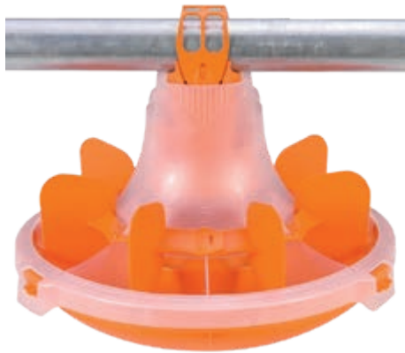
Le dispositif (en option) prévu pour éviter que les poussins ne montent dans le plateau est facile à ajouter ou à retirer.
