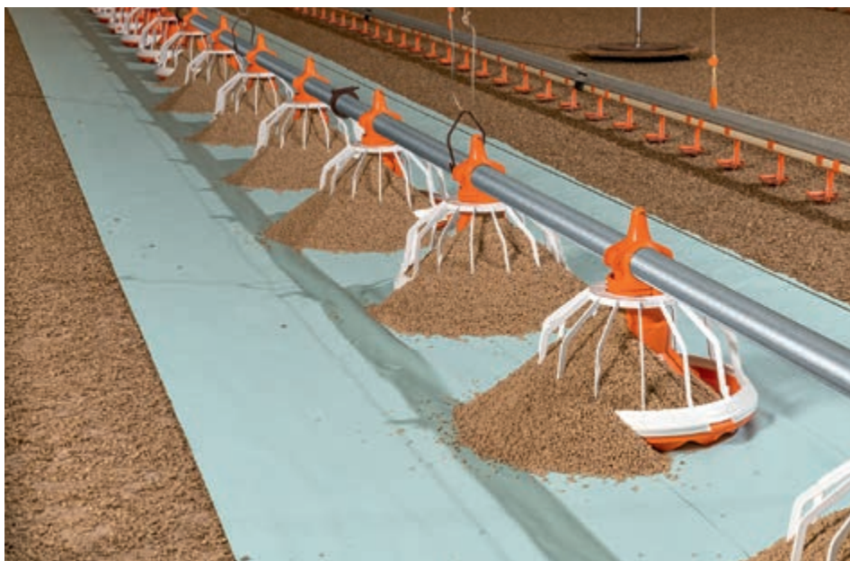
Специално разработената хранилка FLUXX 330 се препълва автоматично за оптимален старт при храненето на едnodневните пилета
