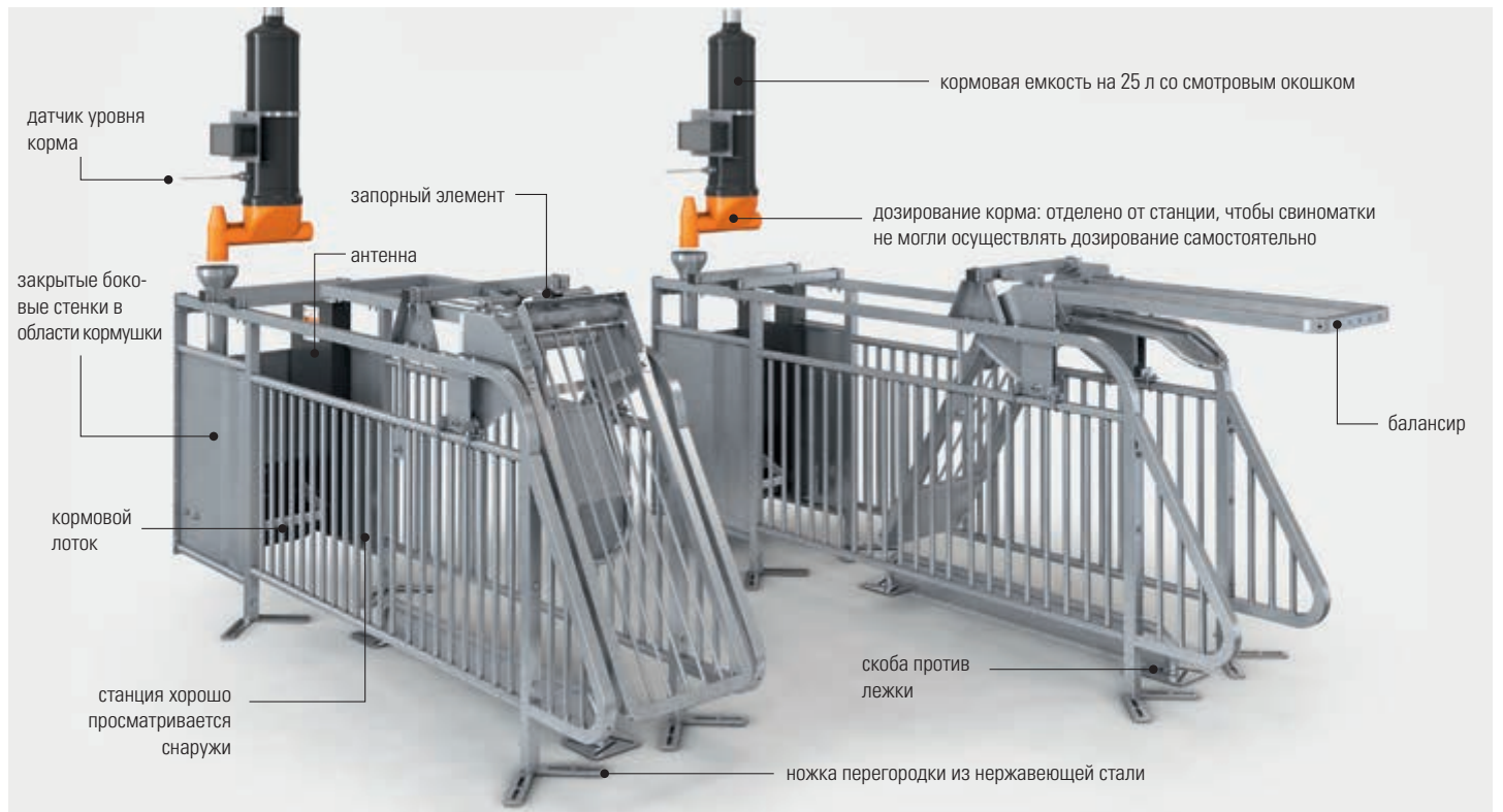
Дозирование корма вручную (опция); кормовая емкость оборудована смотровым окошком для контроля уровня заполнения кормом
