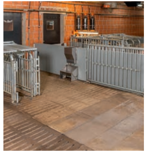
Отдельный интеграционный бокс для свиноматок, позволяющий им легко приобщиться к существующей группе свиноматок; может также использоваться в качестве бокса для больных свиноматок
