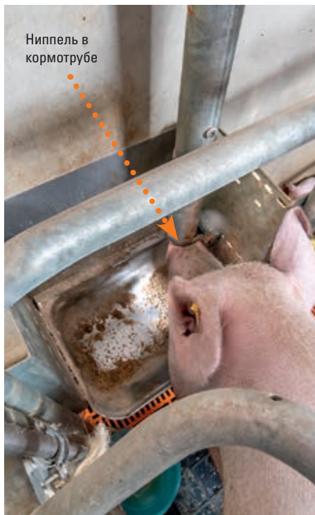
Сенсорное управление: свиноматка приводит в движение ниппель в кормотрубе
