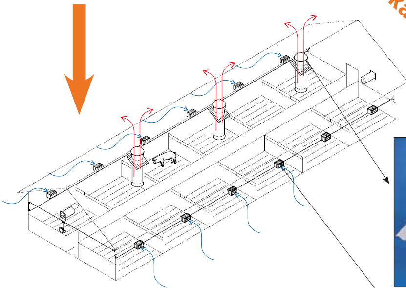
135pro – steruje klimatem w chlewni
