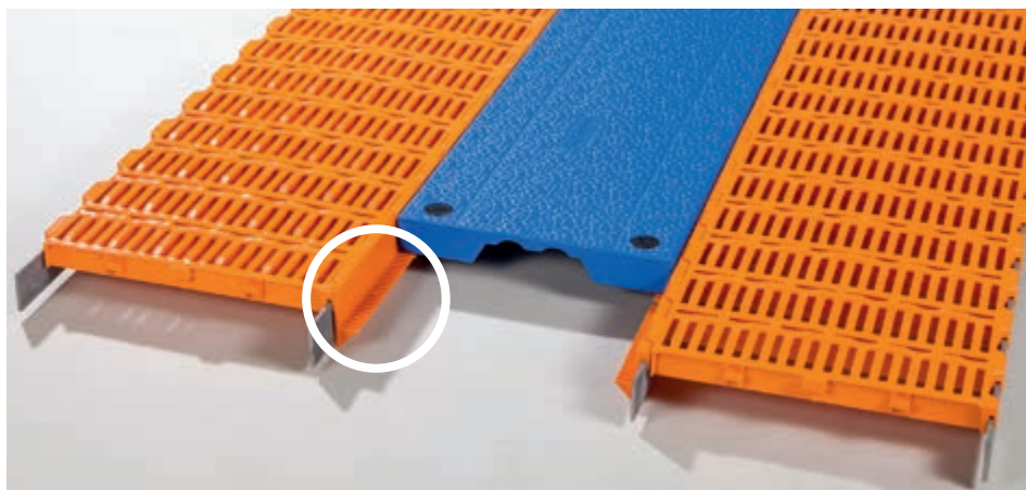
Esempio di montaggio: Semplice assemblaggio dei pannelli riscaldati grazie alle staffe di supporto
