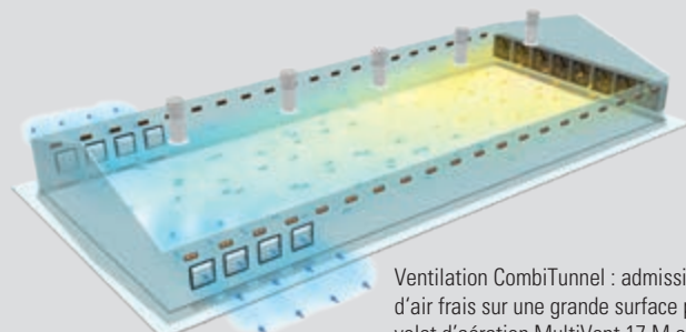
Ventilation CrossTunnel : admission d'air frais sur une grande surface par le volet d'aération MultiVent 10 M, ce qui peut facilement être combiné avec notre système de refroidissement RainMaker
