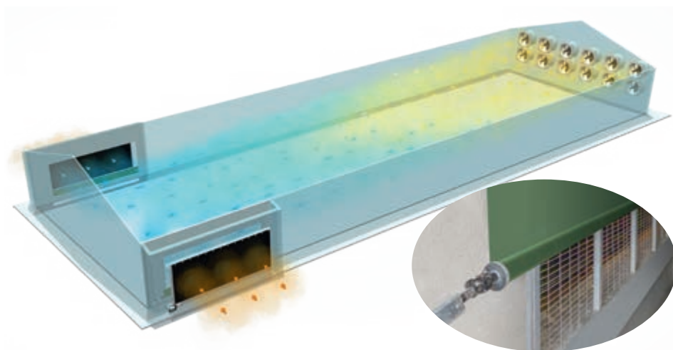
Rideau roulant comme fermeture sûre de tunnel en combinaison avec le système PadCooling RainMaker
