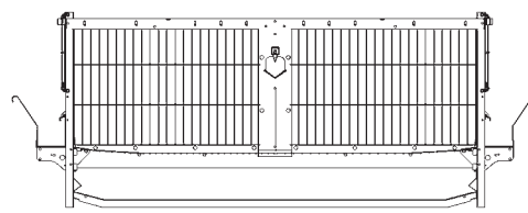
UV-S 680 – ярус для ремонтного молодняка несушек без воздушного канала
