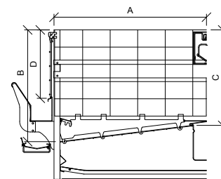
Клетка в разрезе: UV 600a, 600a-plus, 788a с большим воздушным каналом
