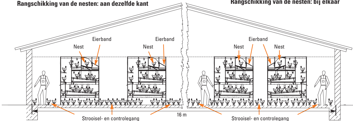
Rangschikking van de nesten: bij elkaar
