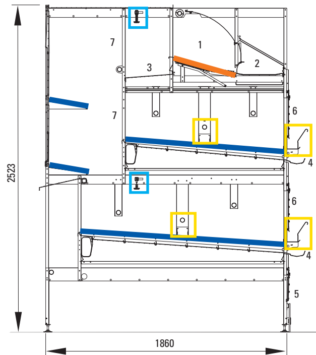
Automatisch openen en sluiten van de afdekking van de eierband (optie)
