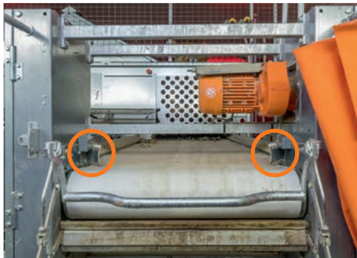
L'avancée rectiligne du tapis est assurée en continu pendant l'opération
